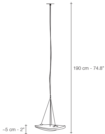
Ø20 cm - 7.9" K011 KK
